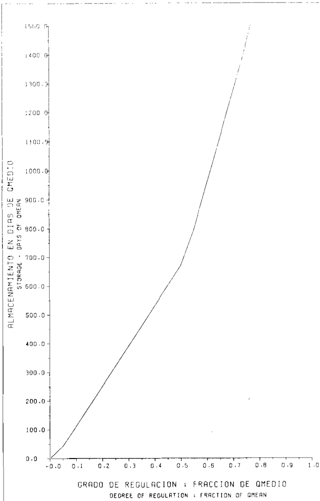
EVALUACION DEL POTENCIAL HIDROELECTRICO NACIONAL CURVA DE ALMACENAMIENTO Y ENTREGA FIRME STORAGE/YIELD CURVE CURVA NO. 203809 Fig. 9-45 A
