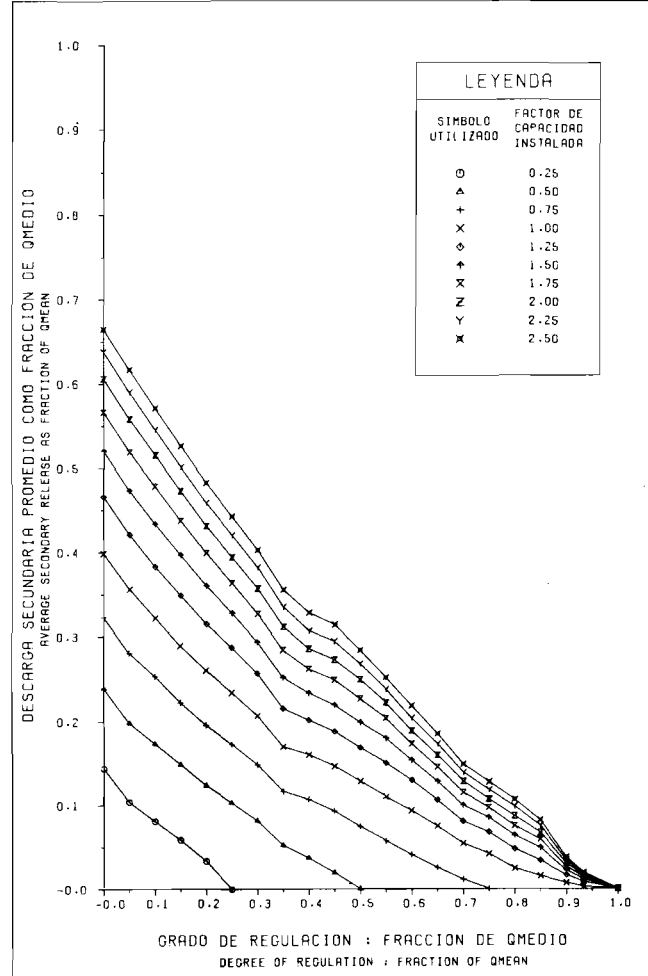
EVALUACION DEL POTENCIAL HIDROELECTRICO NACIONAL CURVAS DE ENTREGA DE RESERVOIR RESERVOIR RELEASE CURVES Fig. 9-46 B CURVA NO. 204001
