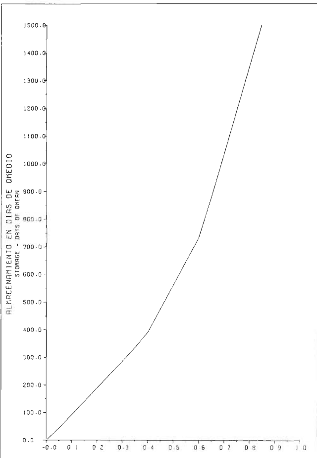
EVALUACION DEL POTENCIAL HIDROELECTRICO NACIONAL CURVA DE ALMACENAMIENTO Y ENTREGA FIRME STORAGE/YIELD CURVE Fig. 9-43 C CURVA NO. 203803
