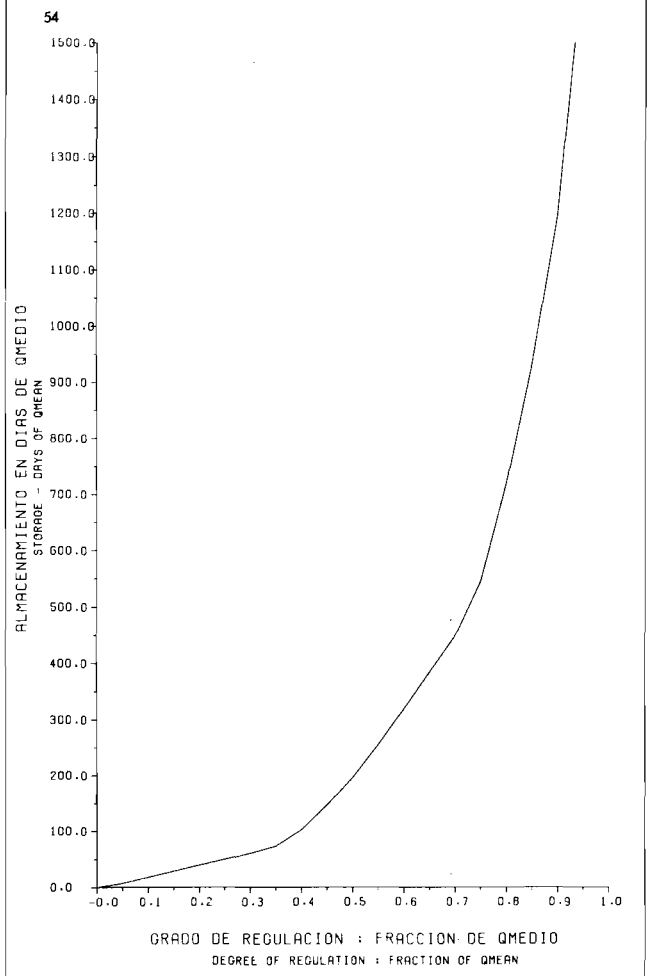
EVALUACION DEL POTENCIAL HIDROELECTRICO NACIONAL CURVA DE ALMACENAMIENTO Y ENTREGA FIRME STORAGE/YIELD CURVE Fig. 9-46 A CURVA NO. 204001
