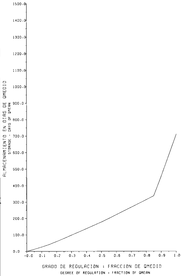
EVALUACION DEL POTENCIAL HIDROELECTRICO NACIONAL CURVA DE ALMACENAMIENTO Y ENTREGA FIRME STORAGE/YIELD CURVE CURVA NO. 202606 Fig. 9-38 A
