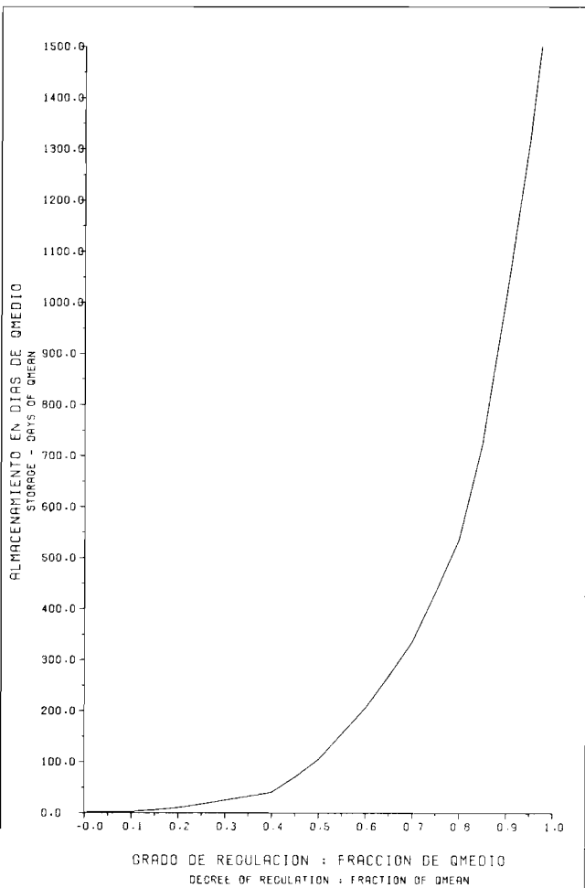
EVALUACION DEL POTENCIAL HIDROELECTRICO NACIONAL CURVA DE ALMACENAMIENTO Y ENTREGA FIRME STORAGE/YIELD CURVE CURVA NO. 202599 Fig. 9-37 C
