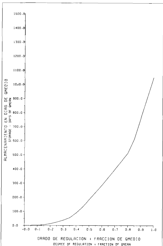
EVALUACION DEL POTENCIAL HIDROELECTRICO NACIONAL CURVAS DE ENTREGA DE RESERVOIRIO RESERVOIR RELEASE CURVES CURVA NO. 204602 Fig. 9-47 D
