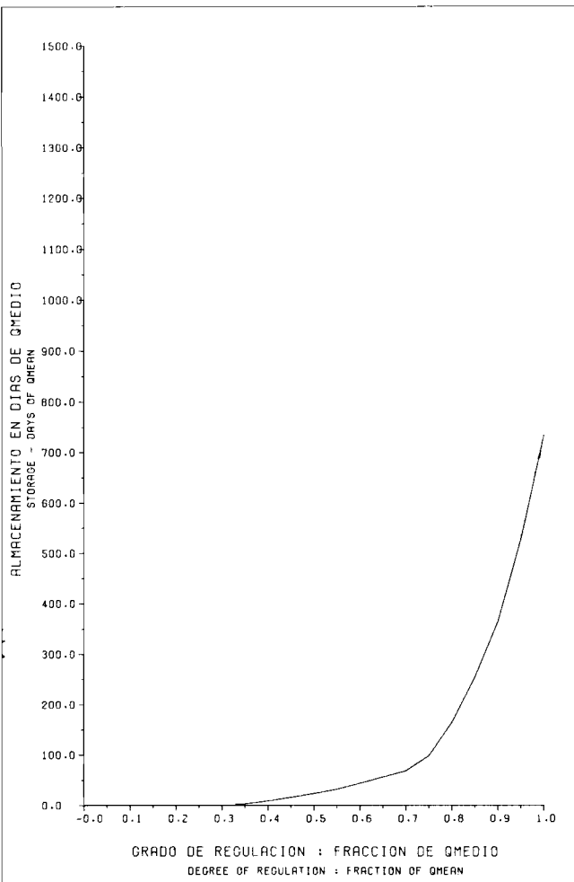
EVALUACION DEL POTENCIAL HIDROELECTRICO NACIONAL CURVA DE ALMACENAMIENTO Y ENTREGA FIRME STORAGE/YIELD CURVE CURVA NO. 202499 Fig. 9-37 A
