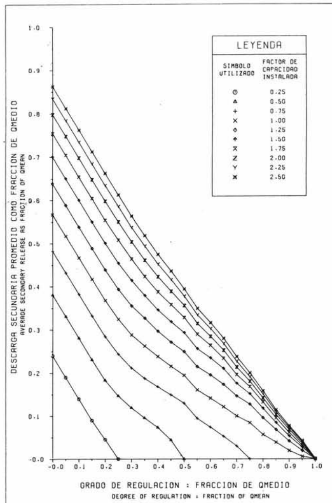
EVALUACION DEL POTENCIAL HIDROELECTRICO NACIONAL CURVAS DE ENTREGA DE RESERVOIR RESERVOIR RELEASE CURVES Fig. 9-42 B CURVA NO. 203399
