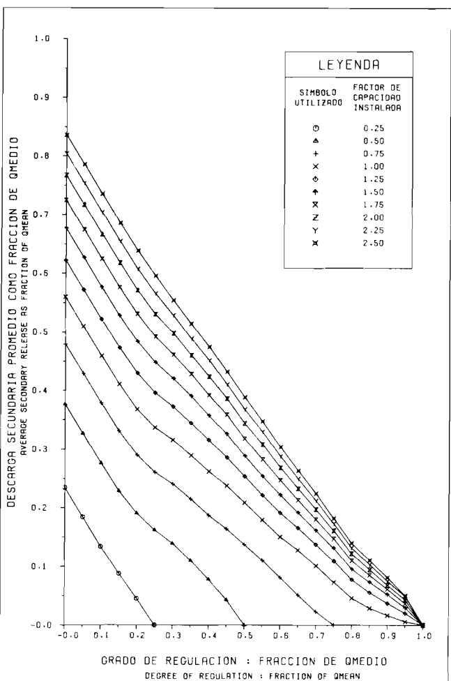
EVALUACION DEL POTENCIAL HIDROELECTRICO NACIONAL CURVA DE ALMACENAMIENTO Y ENTREGA FIRME STORAGE/YIELD CURVE CURVA NO. 204602 Fig. 9-47 C
