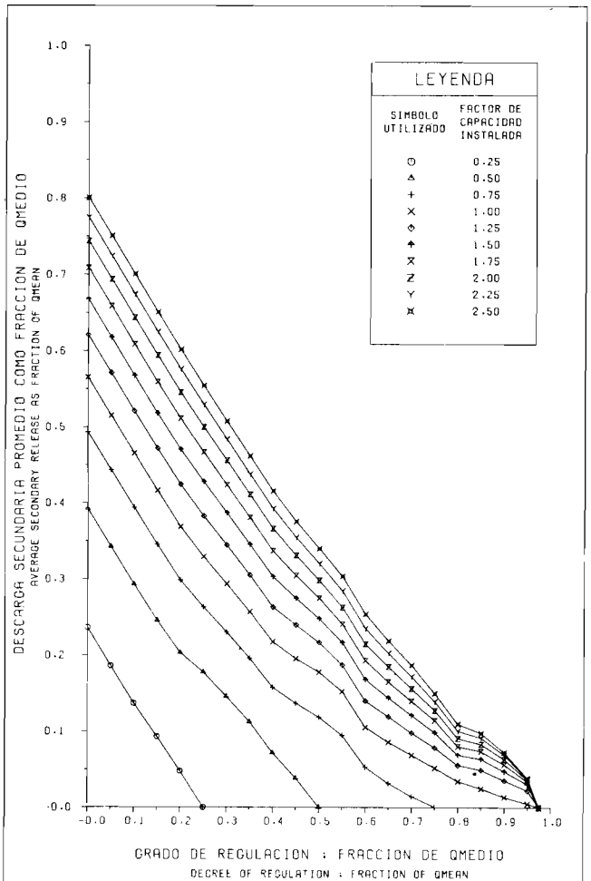
EVALUACION DEL POTENCIAL HIDROELECTRICO NACIONAL CURVAS DE ENTREGA DE RESERVOIR RESERVOIR RELEASE CURVES CURVA NO. 202599 Fig. 9-37 D
