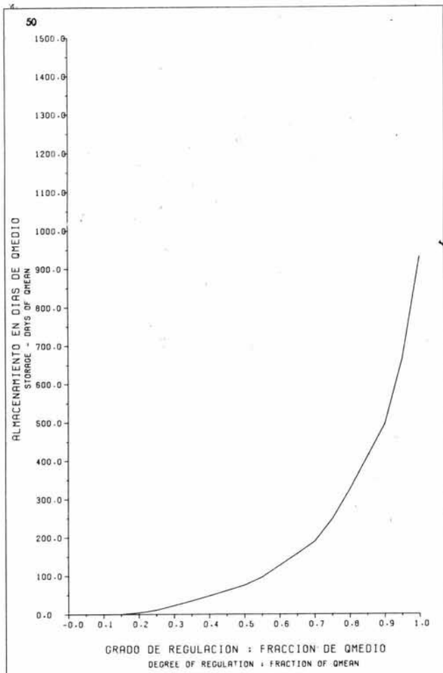
EVALUACION DEL POTENCIAL HIDROELECTRICO NACIONAL CURVA DE ALMACENAMIENTO Y ENTREGA FIRME STORAGE/YIELD CURVE Fig. 9-42 A CURVA NO. 203399
