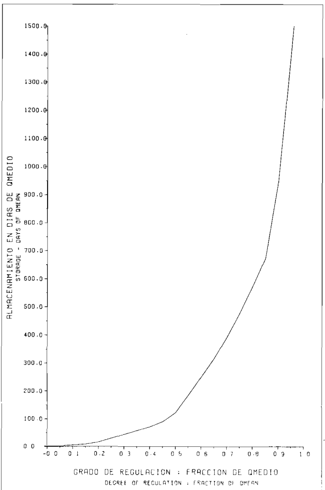
EVALUACION DEL POTENCIAL HIDROELECTRICO NACIONAL CURVA DE ALMACENAMIENTO Y ENTREGA FIRME STORAGE/YIELD CURVE Fig. 9-46 C CURVA NO. 204002
