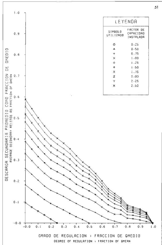
EVALUACION DEL POTENCIAL HIDROELECTRICO NACIONAL CURVAS DE ENTREGA DE RESERVOIR RESERVOIR RELEASE CURVES Fig. 9-43 B CURVA NO. 203799
