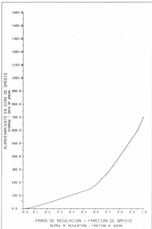
EVALUACION DEL POTENCIAL HIDROELECTRICO NACIONAL CURVA DE ALMACENAMIENTO Y ENTREGA FIRME STORAGE/YIELD CURVE Fig. 9-42 C CURVA NO. 203601
