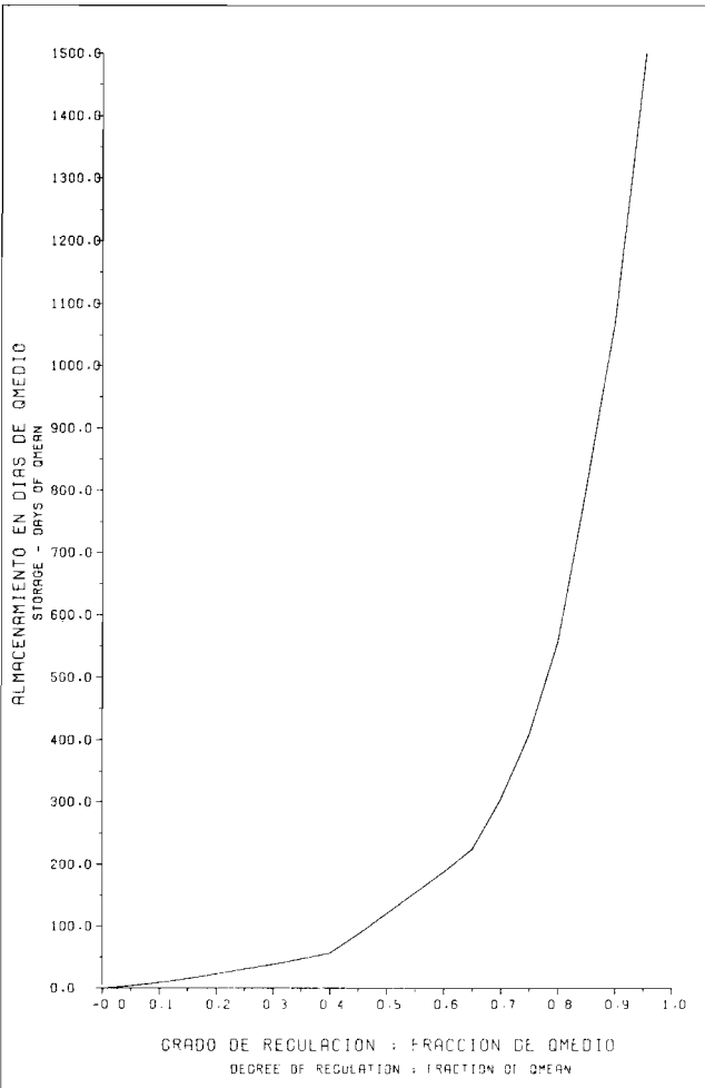
EVALUACION DEL POTENCIAL HIDROELECTRICO NACIONAL CURVA DE ALMACENAMIENTO Y ENTREGA FIRME STORAGE/YIELD CURVE CURVA NO. 202301 Fig. 9-36 C
