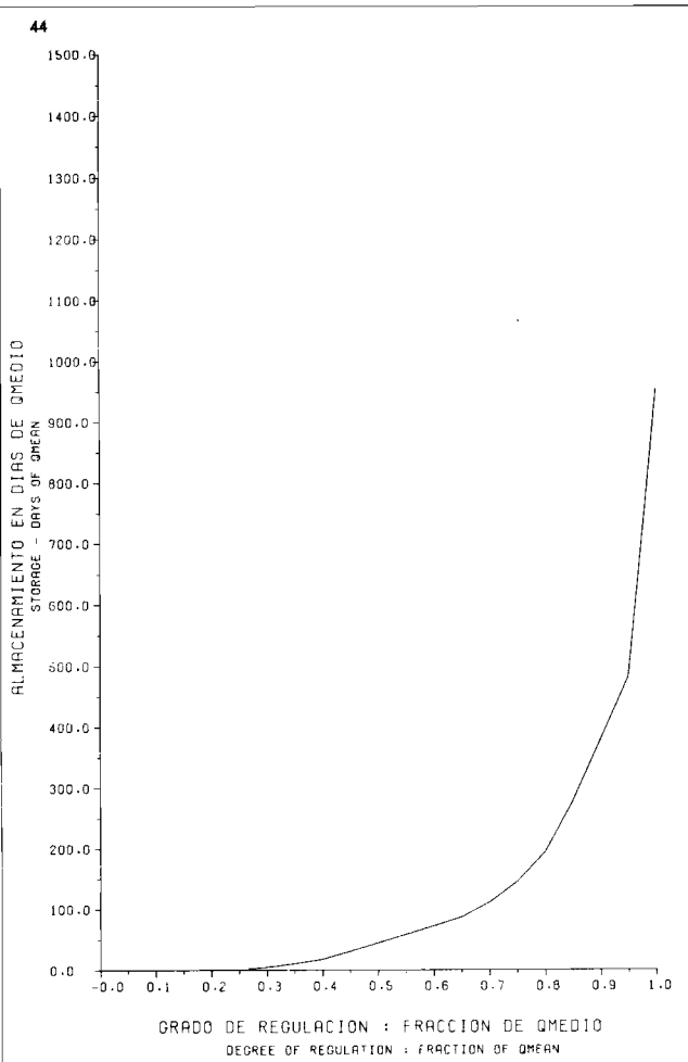
EVALUACION DEL POTENCIAL HIDROELECTRICO NACIONAL CURVA DE ALMACENAMIENTO Y ENTREGA FIRME STORAGE/YIELD CURVE CURVA NO. 201799 Fig. 9-36 A
