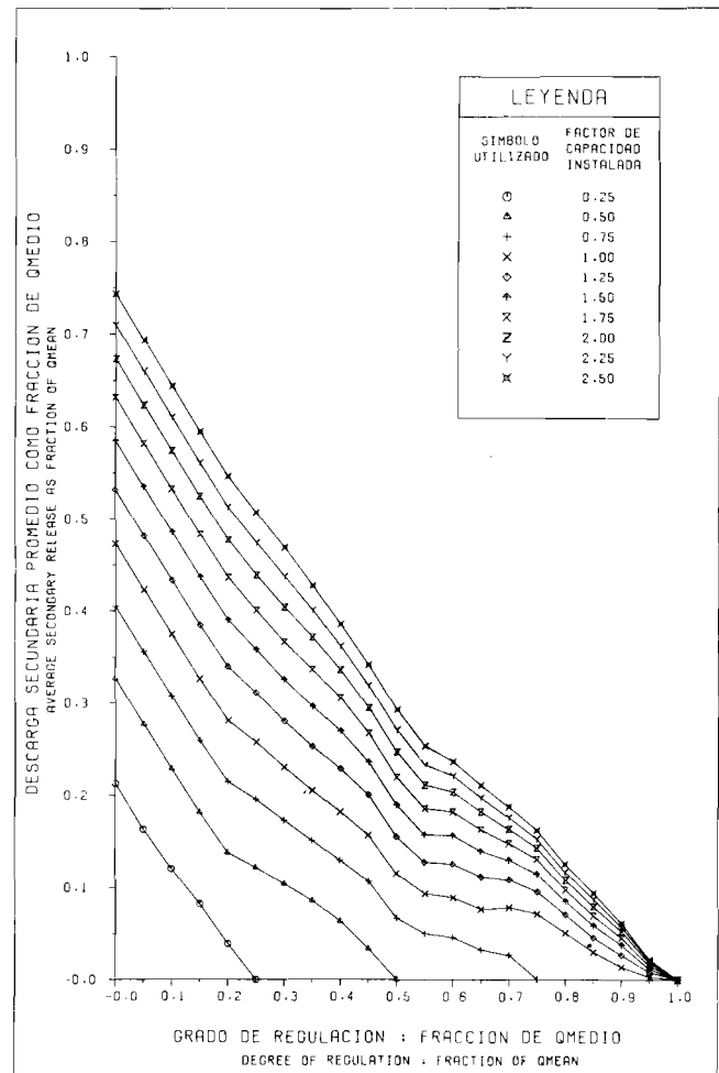
EVALUACION DEL POTENCIAL HIDROELECTRICO NACIONAL CURVAS DE ENTREGA DE RESERVOIR RESERVOIR RELEASE CURVES CURVA NO. 203903 Fig. 9-45 D
