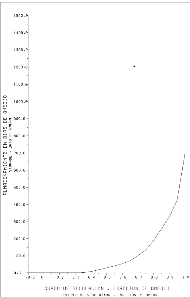
EVALUACION DEL POTENCIAL HIDROELECTRICO NACIONAL CURVA DE ALMACENAMIENTO Y ENTREGA FIRME STORAGE/YIELD CURVE CURVA NO. 202699 Fig. 9-38 C
