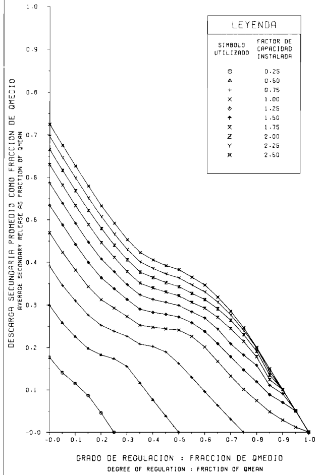
EVALUACION DEL POTENCIAL HIDROELECTRICO NACIONAL CURVAS DE ENTREGA DE RESERVOIR RESERVOIR RELEASE CURVES CURVA NO. 202606 Fig. 9-38 B
