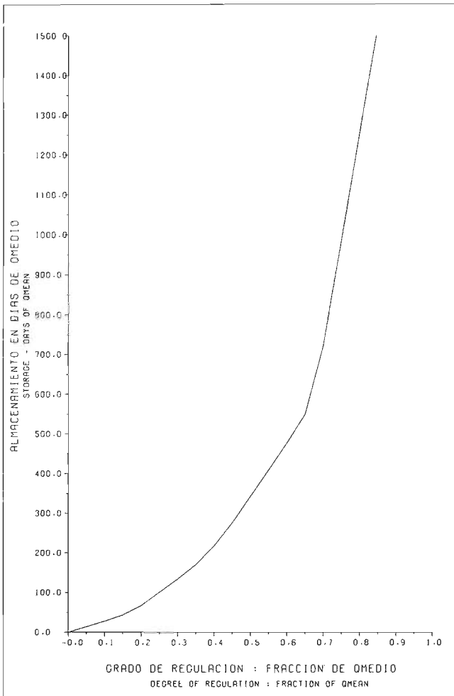
EVALUACION DEL POTENCIAL HIDROELECTRICO NACIONAL CURVA DE ALMACENAMIENTO Y ENTREGA FIRME STORAGE/YIELD CURVE Fig. 9-43 A CURVA NO. 203799
