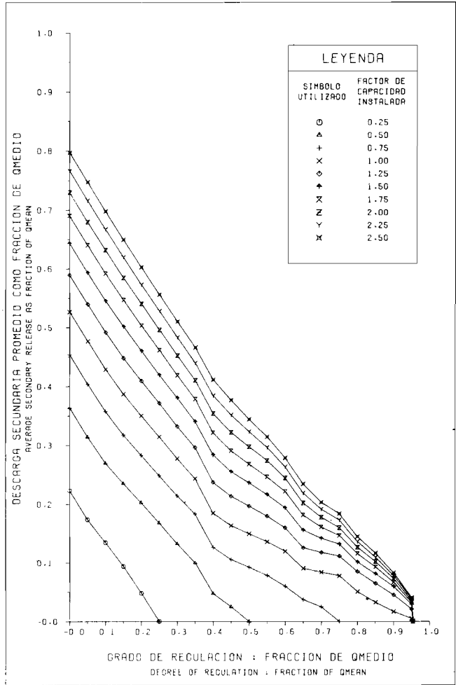
EVALUACION DEL POTENCIAL HIDROELECTRICO NACIONAL CURVAS DE ENTREGA DE RESERVOIRIO RESERVOIR RELEASE CURVES CURVA NO. 202301 Fig. 9-36 D
