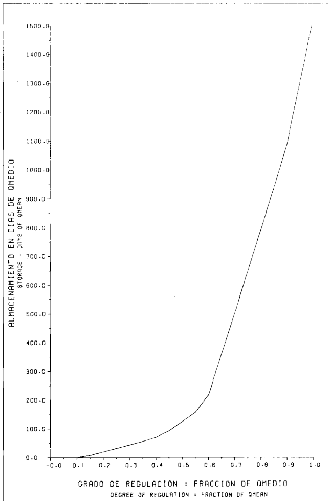
EVALUACION DEL POTENCIAL HIDROELECTRICO NACIONAL CURVA DE ALMACENAMIENTO Y ENTREGA FIRME STORAGE/YIELD CURVE CURVA NO. 204601 Fig. 9-47 A
