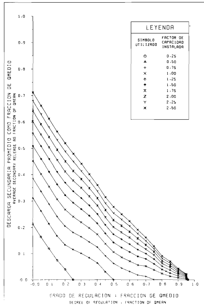
EVALUACION DEL POTENCIAL HIDROELECTRICO NACIONAL CURVAS DE ENTREGA DE RESERVOIR RESERVOIR RELEASE CURVES Fig. 9-46 D CURVA NO. 204002
