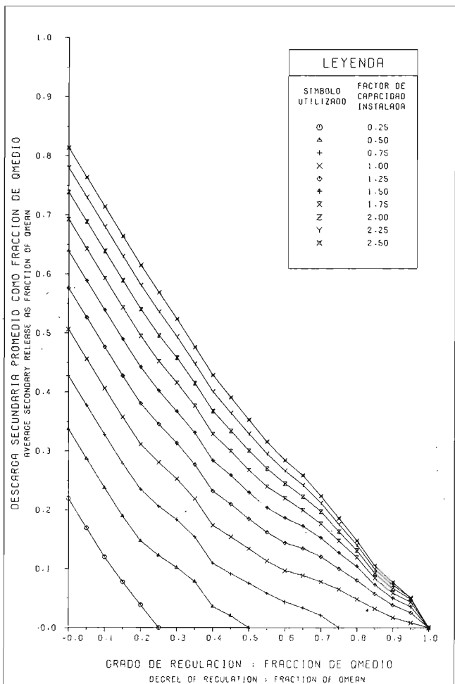
EVALUACION DEL POTENCIAL HIDROELECTRICO NACIONAL CURVAS DE ENTREGA DE RESERVOIRIO RESERVOIR RELEASE CURVES Fig. 9-41 D CURVA NO. 203199
