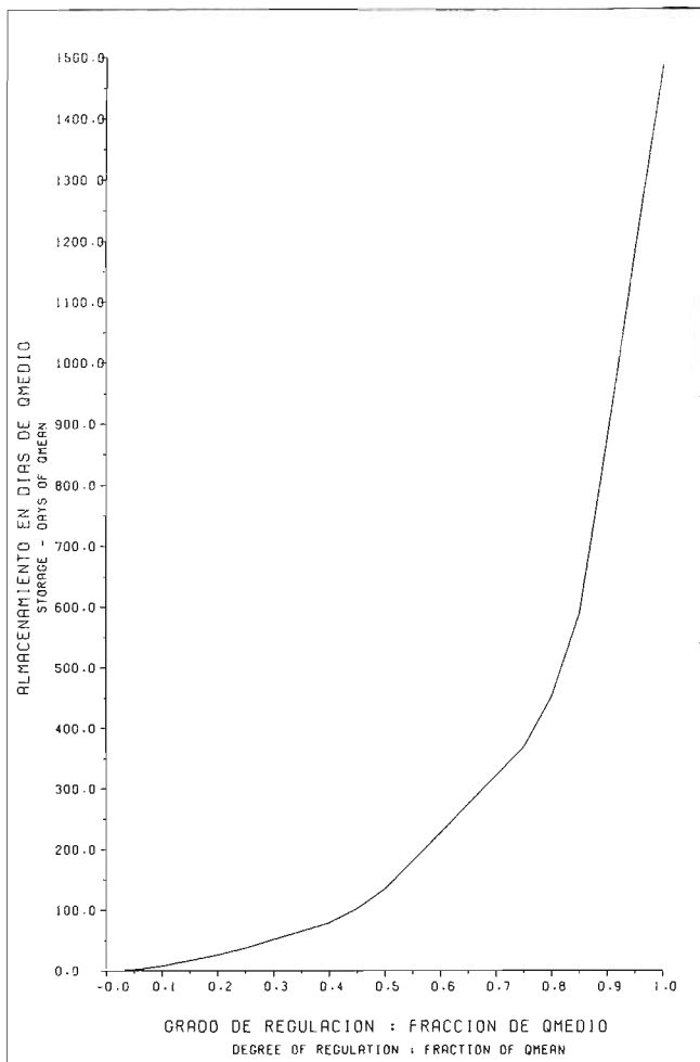
EVALUACION DEL POTENCIAL HIDROELECTRICO NACIONAL CURVA DE ALMACENAMIENTO Y ENTREGA FIRME STORAGE/YIELD CURVE Fig. 9-41 A CURVA NO. 203001
