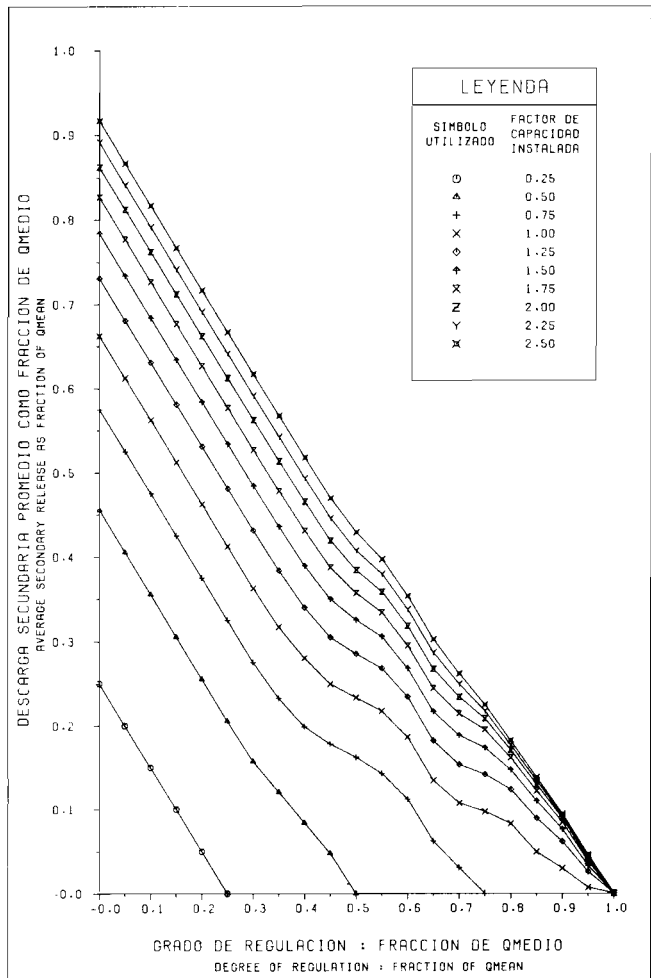
EVALUACION DEL POTENCIAL HIDROELECTRICO NACIONAL CURVAS DE ENTREGA DE RESERVOIRIO RESERVOIR RELEASE CURVES CURVA NO. 201799 Fig. 9-36 B
