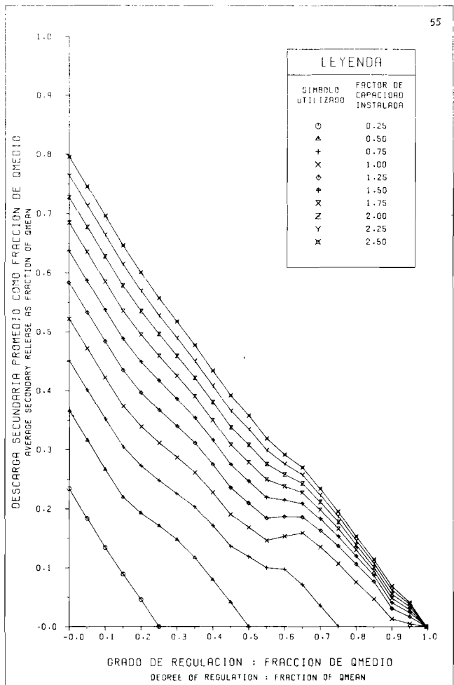
EVALUACION DEL POTENCIAL HIDROELECTRICO NACIONAL CURVAS DE ENTREGA DE RESERVOIRIO RESERVOIR RELEASE CURVES CURVA NO. 204601 Fig. 9-47 B
