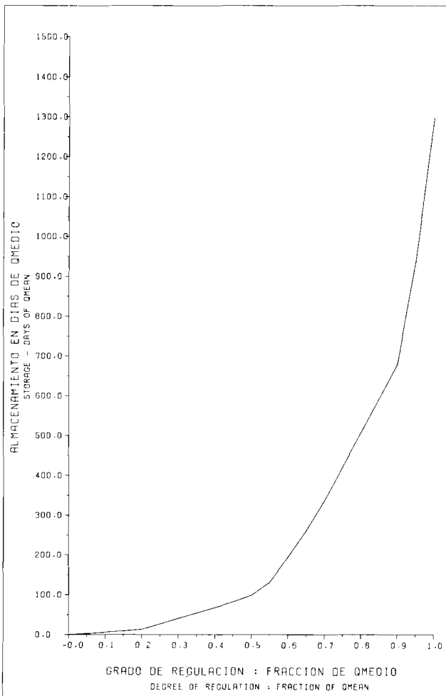
EVALUACION DEL POTENCIAL HIDROELECTRICO NACIONAL CURVA DE ALMACENAMIENTO Y ENTREGA FIRME STORAGE/YIELD CURVE CURVA NO. 203903 Fig. 9-45 C
