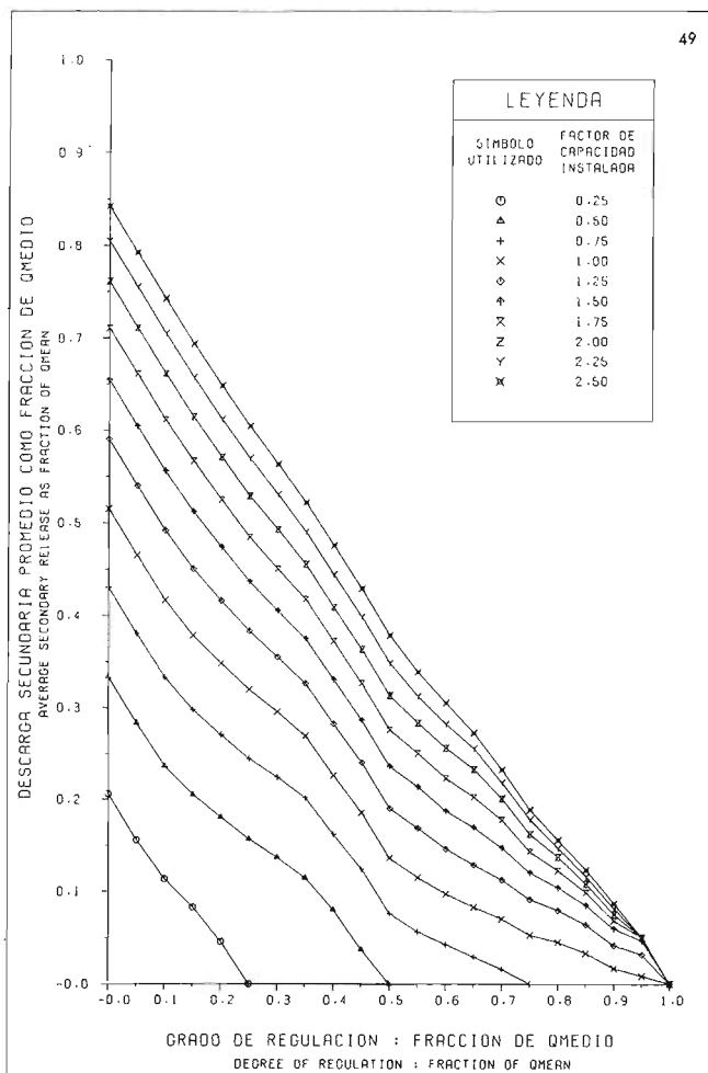
EVALUACION DEL POTENCIAL HIDROELECTRICO NACIONAL CURVAS DE ENTREGA DE RESERVOIRIO RESERVOIR RELEASE CURVES Fig. 9-41 B CURVA NO. 203001
