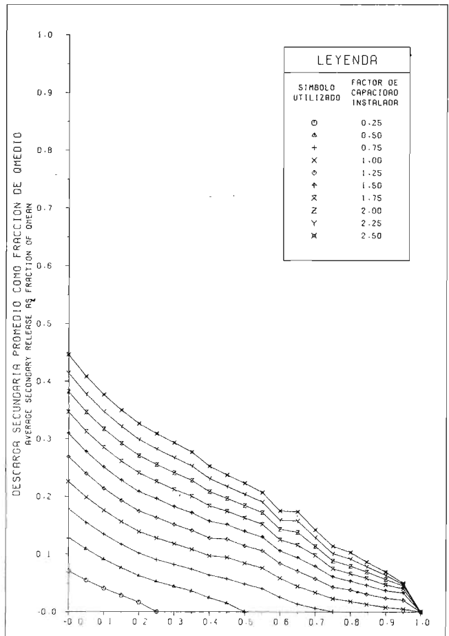
EVALUACION DEL POTENCIAL HIDROELECTRICO NACIONAL CURVAS DE ENTREGA DE RESERVOIR RESERVOIR RELEASE CURVES Fig. 9-43 D CURVA NO. 203803
