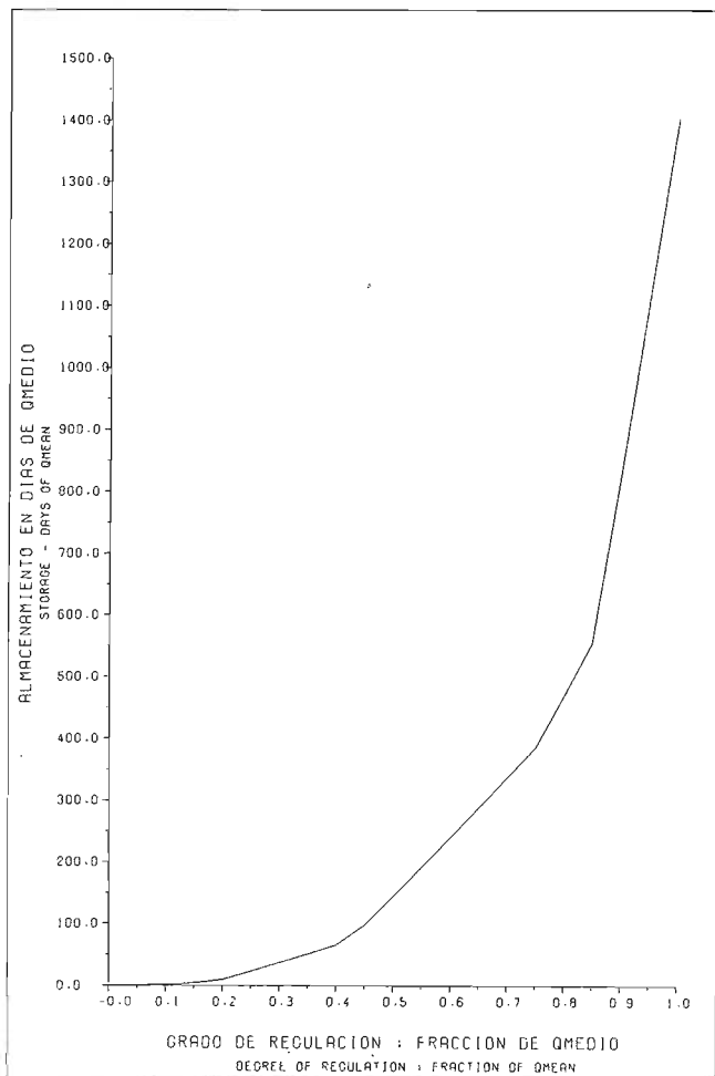
EVALUACION DEL POTENCIAL HIDROELECTRICO NACIONAL CURVA DE ALMACENAMIENTO Y ENTREGA FIRME STORAGE/YIELD CURVE Fig. 9-41 C CURVA NO. 203199
