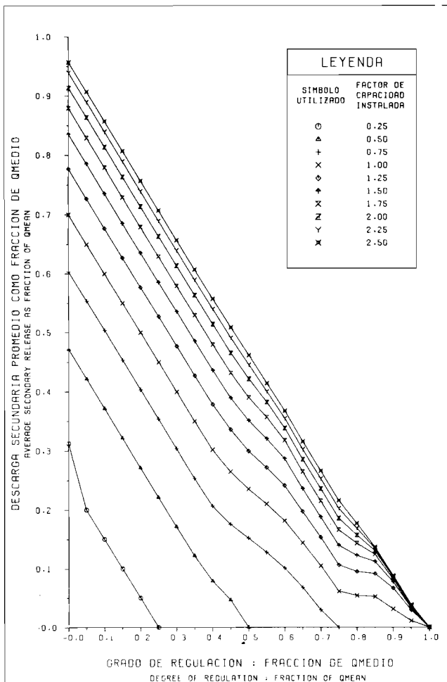
EVALUACION DEL POTENCIAL HIDROELECTRICO NACIONAL CURVAS DE ENTREGA DE RESERVOIR RESERVOIR RELEASE CURVES CURVA NO. 202699 Fig. 9-38 D
