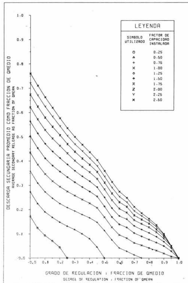
EVALUACION DEL POTENCIAL HIDROELECTRICO NACIONAL CURVAS DE ENTREGA DE RESERVOIR RESERVOIR RELEASE CURVES Fig. 9-42 D CURVA NO. 203601
