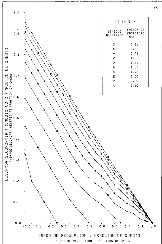
EVALUACION DEL POTENCIAL HIDROELECTRICO NACIONAL CURVAS DE ENTREGA DE RESERVOIR RESERVOIR RELEASE CURVES CURVA NO. 202499 Fig. 9-37 B
