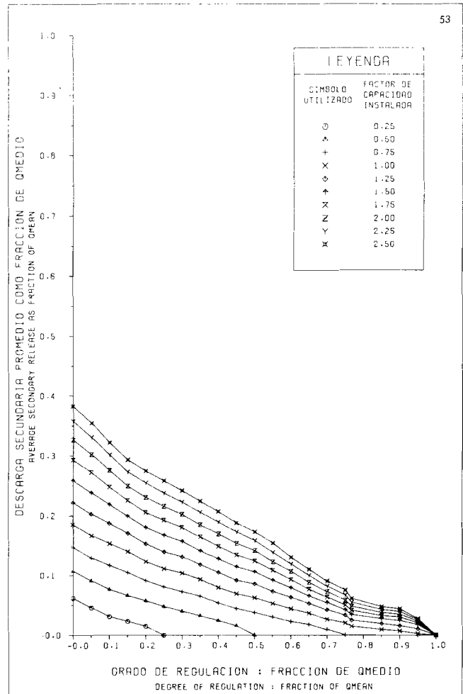
EVALUACION DEL POTENCIAL HIDROELECTRICO NACIONAL CURVAS DE ENTREGA DE RESERVOIR RESERVOIR RELEASE CURVES CURVA NO. 203809 Fig. 9-45 B
